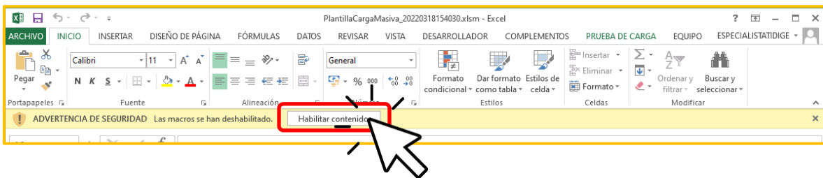
Figura 27. Archivo Excel.
