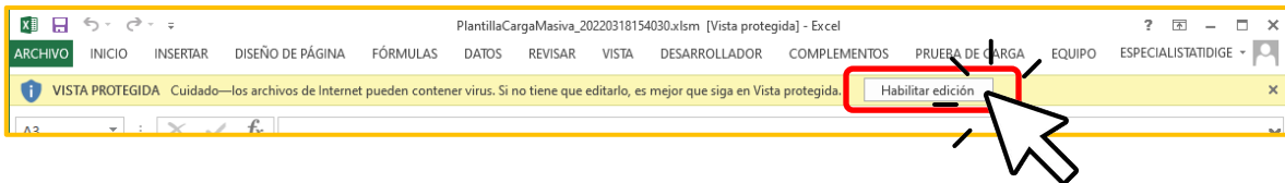
Figura 26. Archivo Excel.
